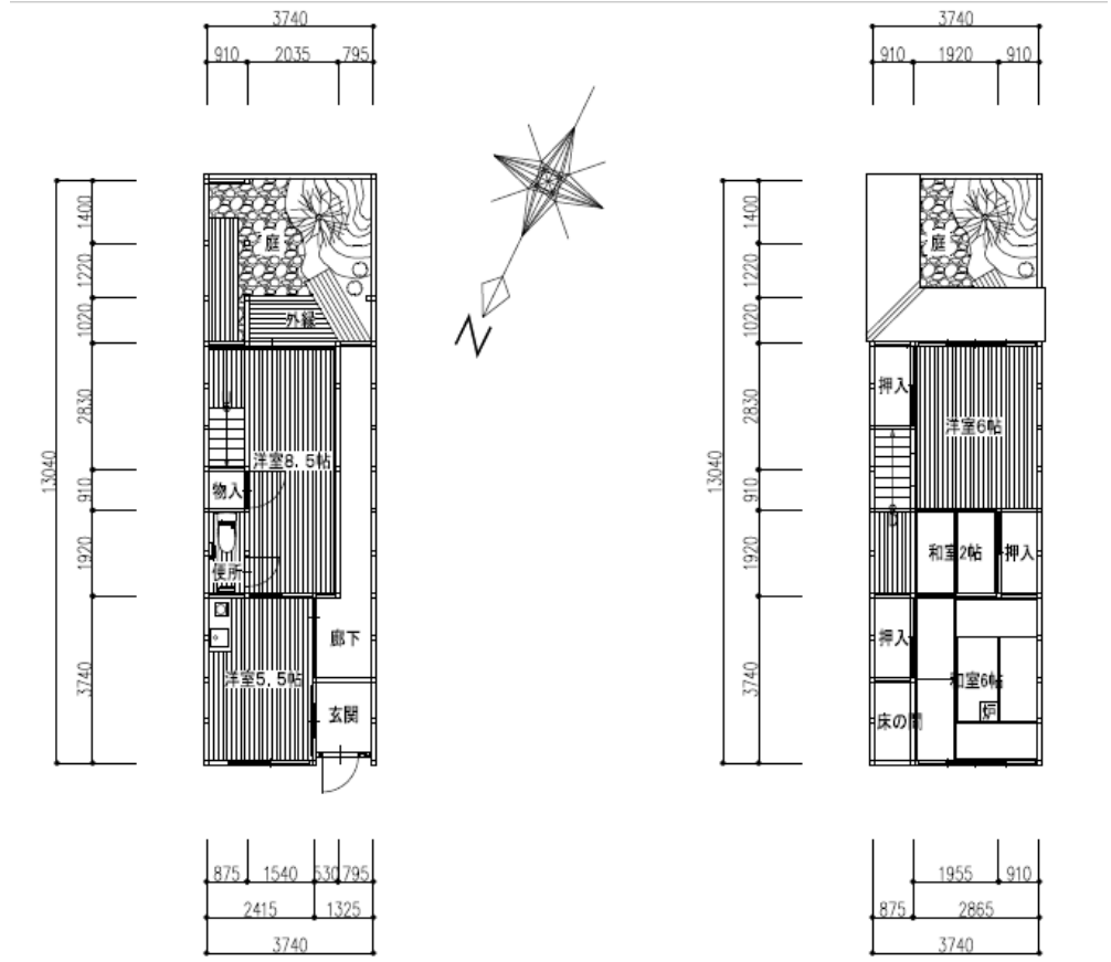
1階平面図 1/100
