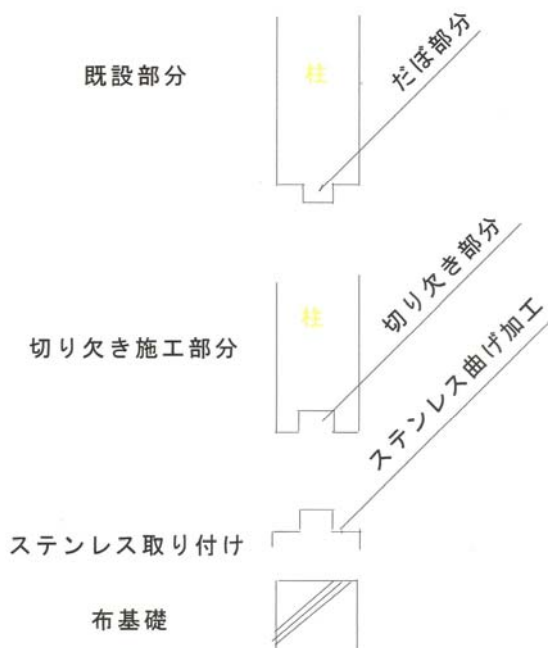
柱脚部修復概説図
