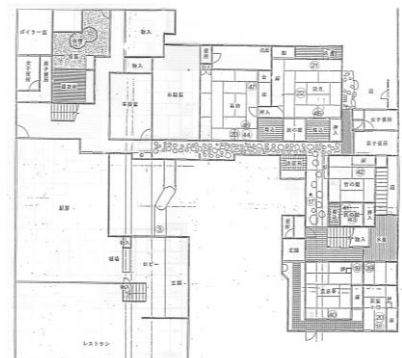
1階平面図
